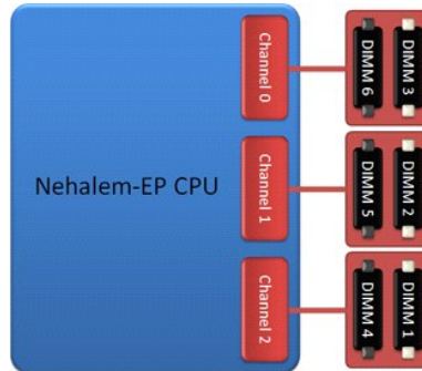
Konfigurasi slot DIMM untuk prosesor tunggal atau prosesor kedua pada riser.
