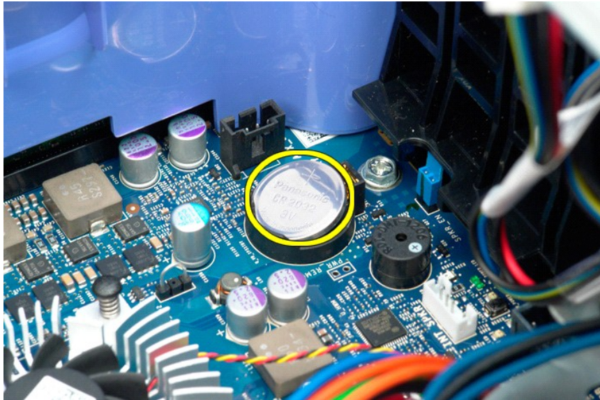
4. Lepaskan sel berbentuk koin dari komputer.
