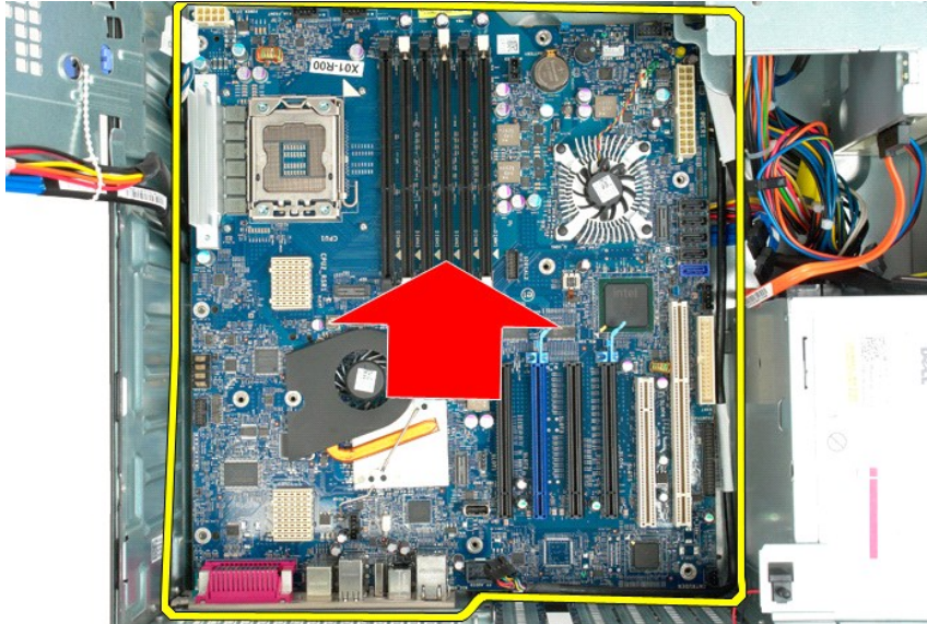
19. Lepaskan board sistem.
